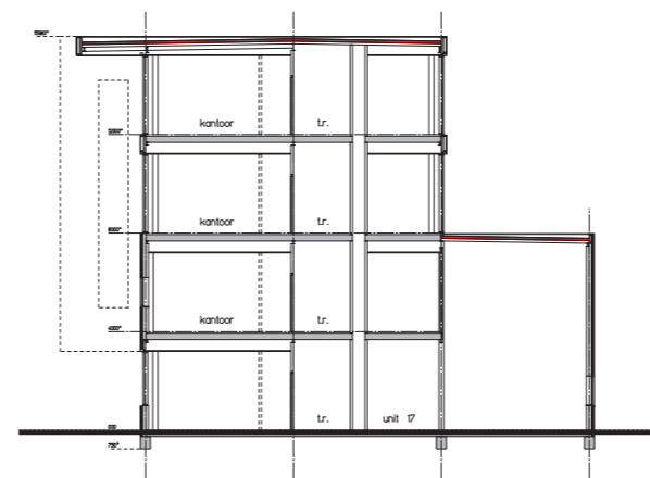
DOORSNEDE EE
