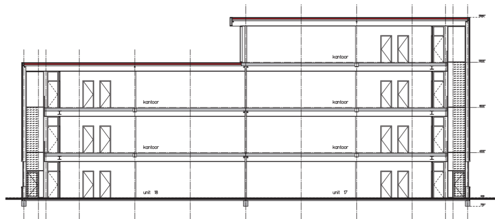
DOORSNEDE DD
