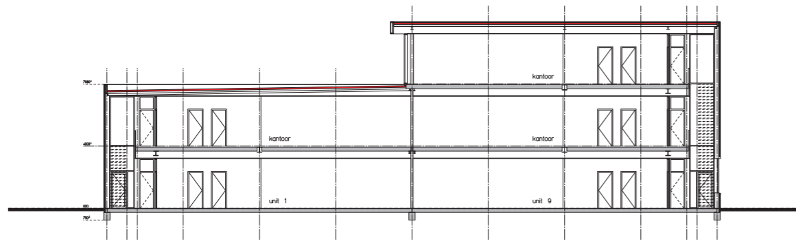
DOORSNEDE BB
